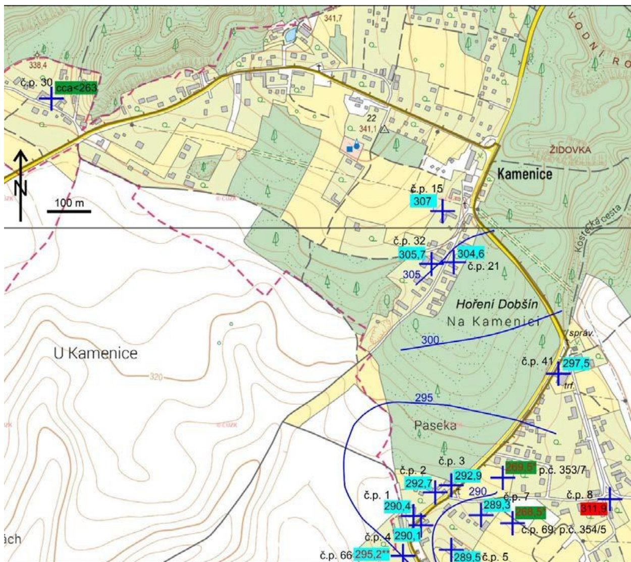
Obr. 5. Nadmořské výšky hladin podzemní vody (m n. m.) v jednotlivých zvodnících v Dobšíně v období 15.–21.2.2024.
